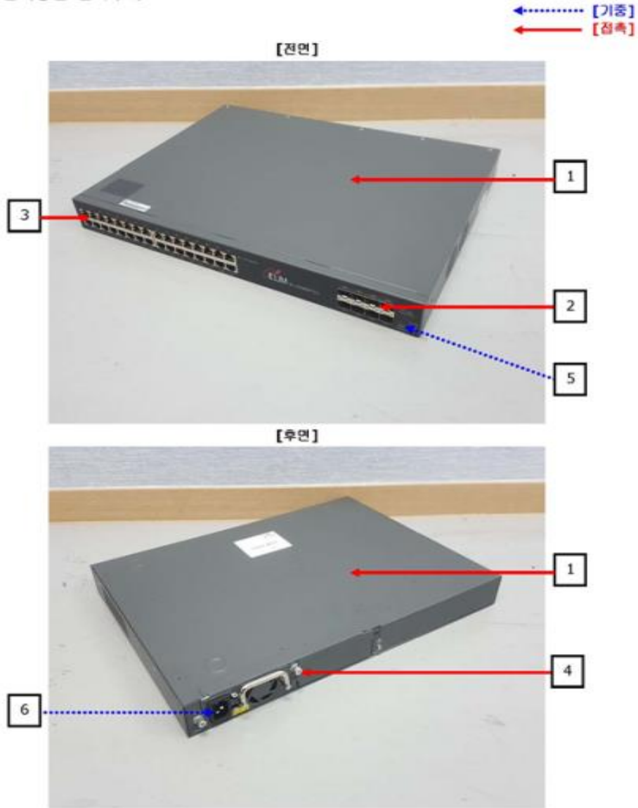
정전기방전 인가부위
