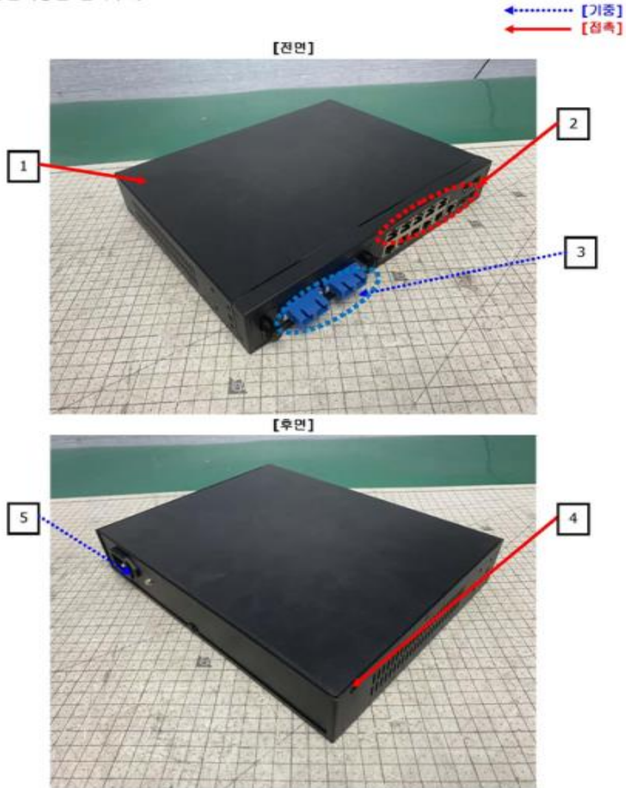
정전기방전 인가부위
